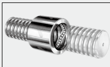
圖3.2 內循環滾珠螺桿
