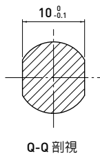
Q-Q 剖視
