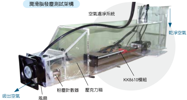
潤滑脂發塵測試架構
